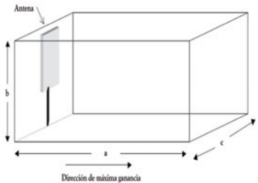
Figura 5. Paralelepípedo de protección
