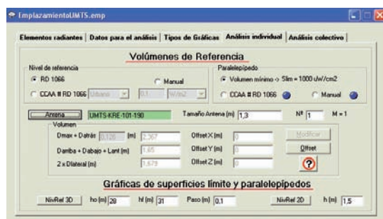
Figura 54. Análisis individual de las antenas UMTS
