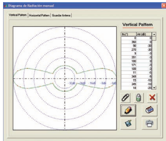
Figura 61 A. Diagramas de radiación vertical de la antena de Radiodifusión FM
