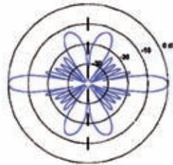
Figura 21. Diagrama de radiación normalizado
