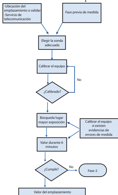
Figura 40. Fase-1 de medidas
