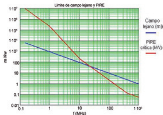
Figura 19. Relación entre PIRE crítica y campo lejano
