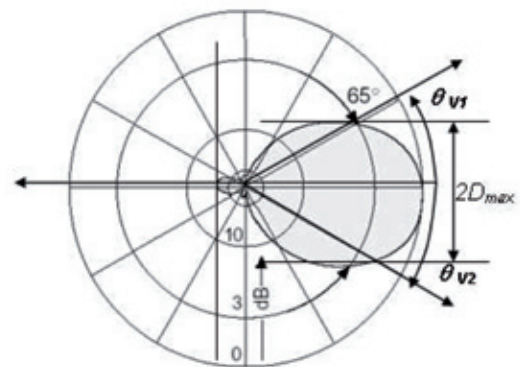
Figura 45. Diagrama de radiación vertical
