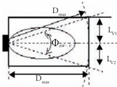
Figura 12. Cálculo del paralelepípedo de referencia (vista superior)
