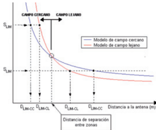
Figura 11. Comparación de los modelos de campo cercano y campo lejano
