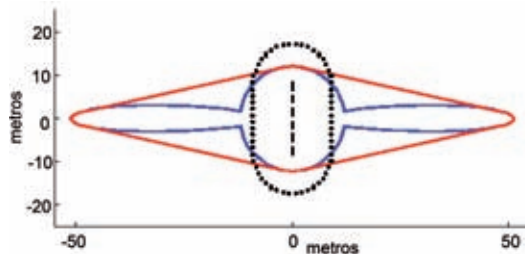
Figura 26. Superficie de protección calculada a partir del diagrama de radiación simulado
