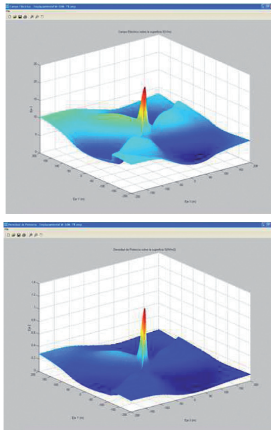
Figura 64. Densidad de Potencia y Campo Eléctrico en el Emplazamiento
