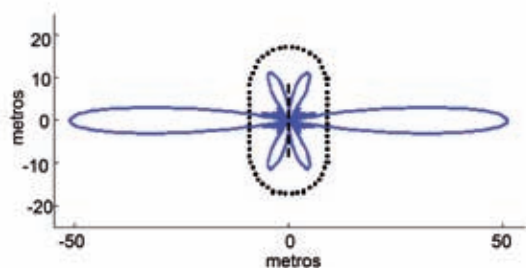
Figura 23. Superficie de protección: campo lejano
