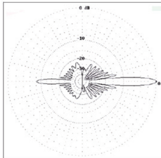
Figura 30. Diagrama de radiación de la agrupación de dipolos (dB). Plano vertical
