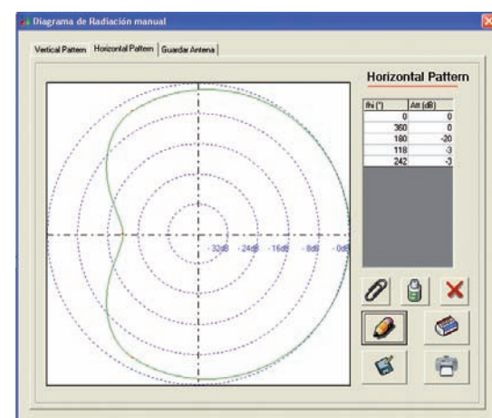
Figura 59. Diagramas de radiación vertical y horizontal de antenas de Televisión tipo 1
