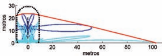
Figura 29. Superficie de protección corregida
