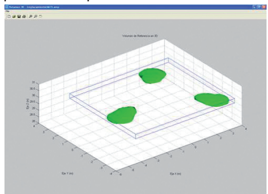
Figura 57. Paralelepípedo de referencia del emplazamiento y las antenas propuestas resultante del análisis colectivo de los elementos radiantes
