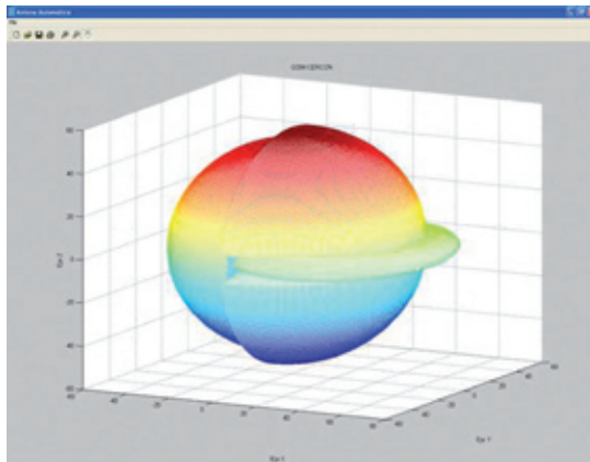
Figura 62. Diagramas de radiación 3D de las antenas de Telefonía Móvil GSM
