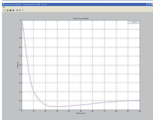
Figura 66. Perfil de Accesibilidad para Ángulos de 113°, 120°, 140°, 174° y 215°
