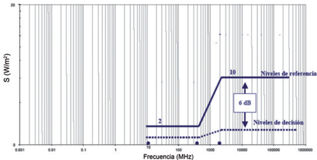
Figura 3. Niveles de referencia y de decisión. Densidad de Potencia
