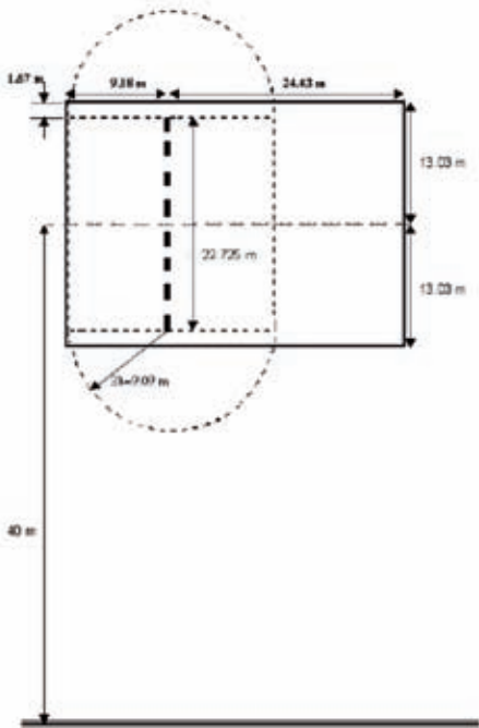
Figura 31. Paralelepípedo de referencia para el sistema considerado
