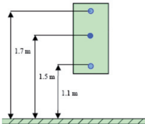
Figura 39. Elección de los puntos de medida.
