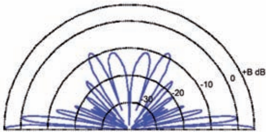
Figura 28. Diagrama de radiación corregido por el efecto del suelo
