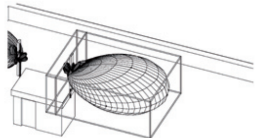
Figura 10. Situación del paralelepípedo de referencia
