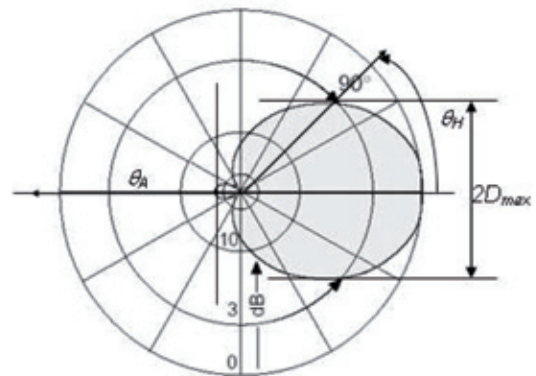
Figura 44. Diagrama de radiación horizontal
