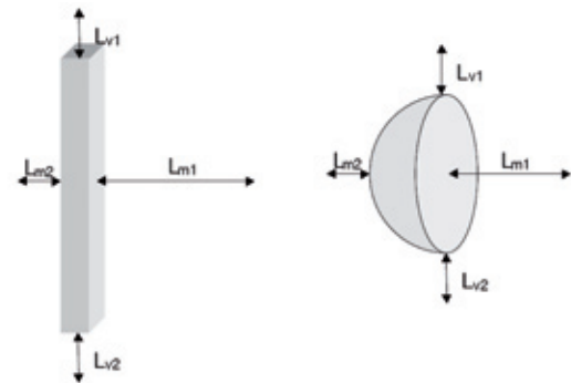
Figura 9. Dimensiones del paralelepípedo de referencia para dos antenas distintas
