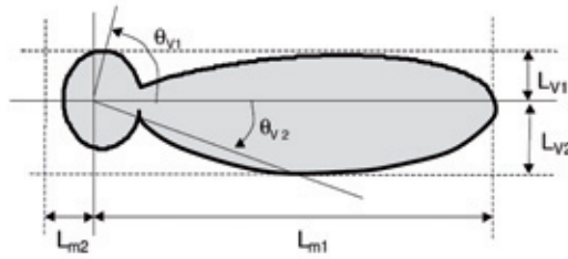
Figura 8. Cálculo del paralelepípedo de referencia a partir del diagrama de radiación de la antena. (Diagramas de campo normalizado en unidades naturales)
