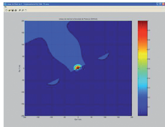
Figura 65 B. Líneas de Nivel de Campo Eléctrico en el Emplazamiento para una altura sobre la azotea de 2 metros
