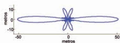
Figura 22. Superficie de protección centrada en la agrupación de dipolos
