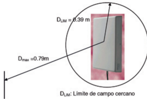
Figura 42. Distancia de referencia y límite de campo cercano
