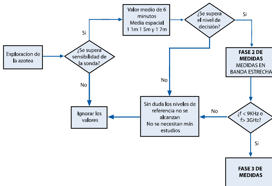
Figura 4. Protocolo de medidas. Diagrama de flujo
