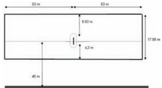
Figura 35. Paralelepípedo de referencia para el sistema radiante considerado
