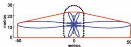
Figura 27. Superficie de protección: estimación del efecto del suelo
