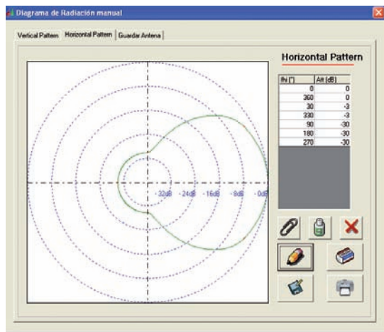
Figura 60. Diagramas de radiación vertical y horizontal de la antena de Televisión tipo 2
