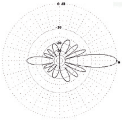
Figura 32. Diagrama de radiación de la agrupación de dipolos (dB). Plano vertical
