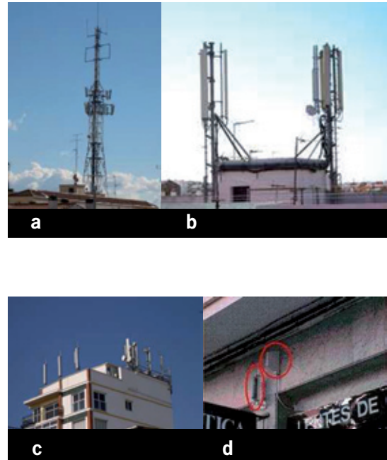
Figura 36. Ejemplos de antenas de telefonía móvil
