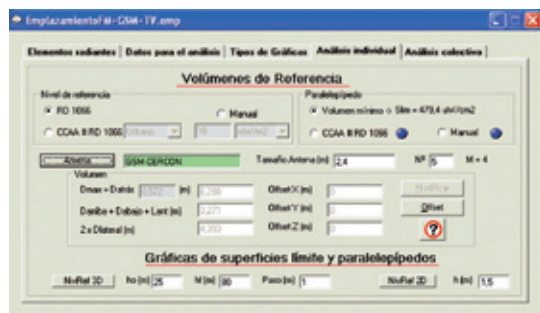
Figura 71. Análisis individual de la antena de Telefonía Móvil GSM Nº1
