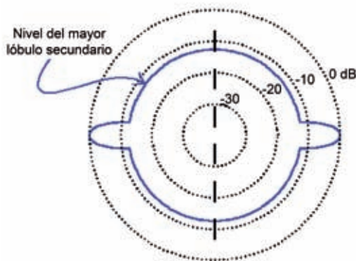
Figura 25. Diagrama de radiación simulado a partir del lóbulo principal
