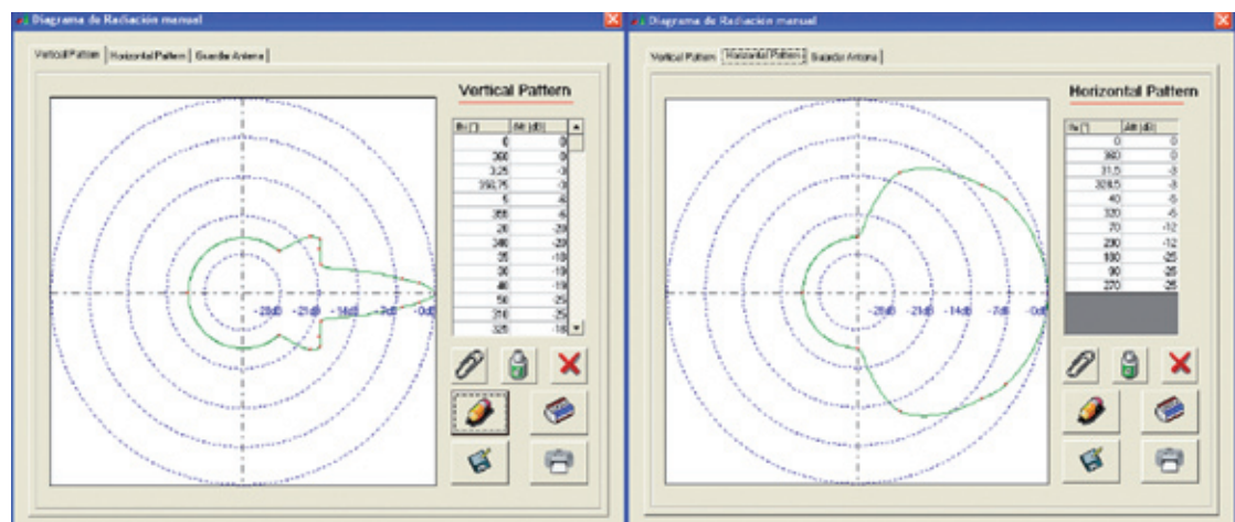
Figura 49. Diagramas de radiación vertical y horizontal de la antena UMTS
