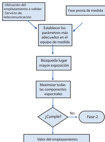
Figura 41. Fase-2 de medidas
