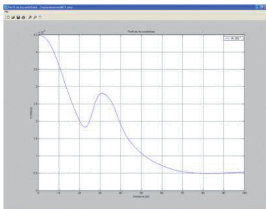
Figura 53C. Perfil de Accesibilidad para Ángulo de 350º
