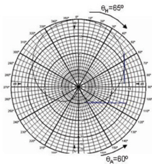
Figura 16. Diagramas de radiación (valores de campo en dB)
