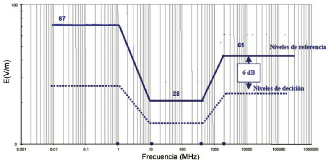
Figura 2. Niveles de referencia y de decisión. Intensidad de campo eléctrico
