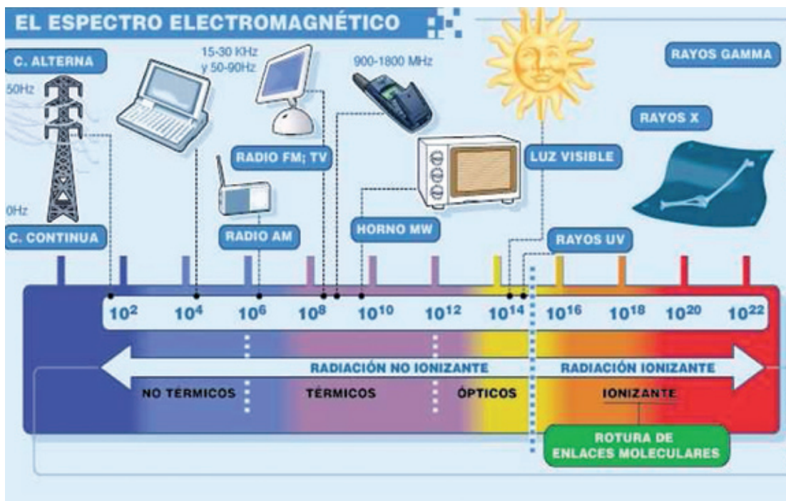
Figura 1. El espectro electromagnético.
