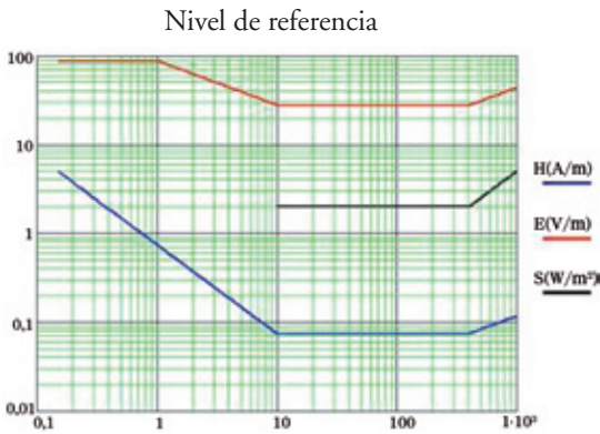
Figura 18. Niveles de referencia de campo eléctrico, magnético y densidad de potencia
