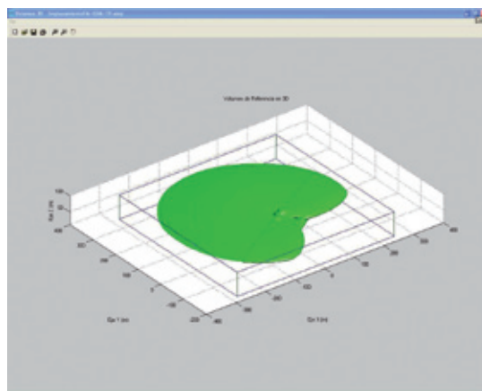
Figura 75. Paralelepípedo de referencia del emplazamiento y las antenas propuestas resultante del análisis colectivo de los elementos radiantes
